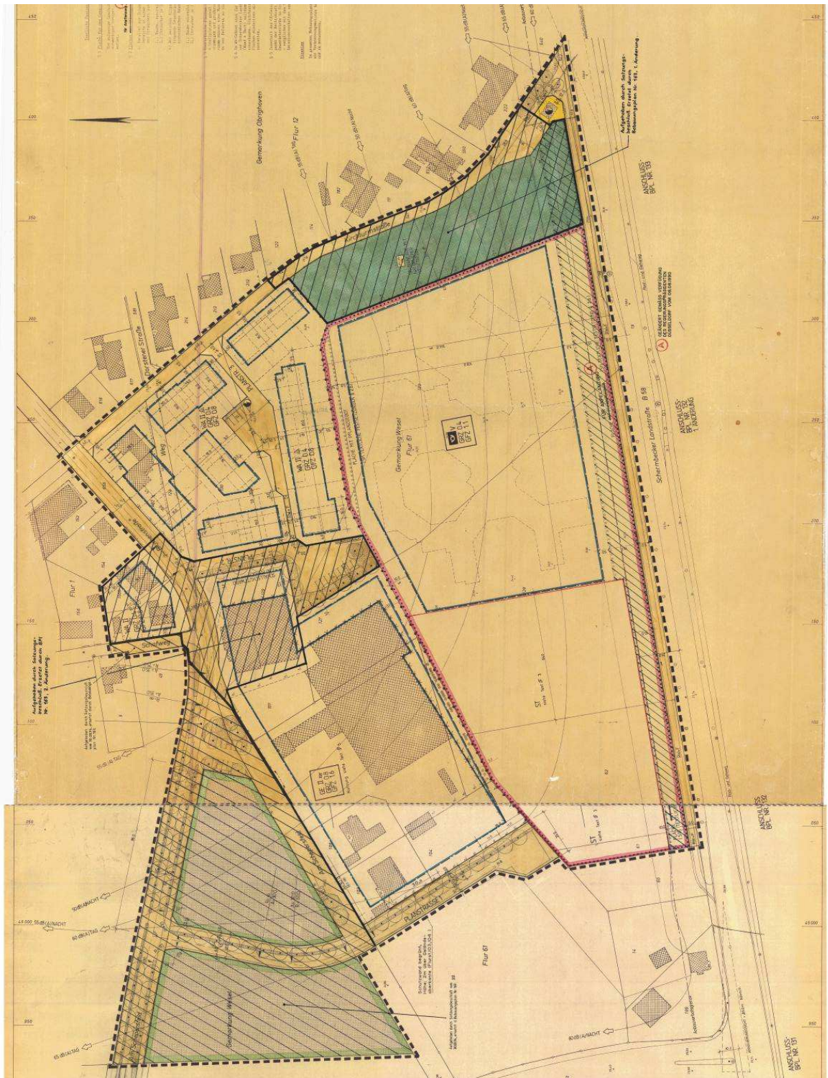
Bebauungsplan Nr. 163 "Am Regnit", Vereinfachte Änderung A derzeitiges Planungsrecht
